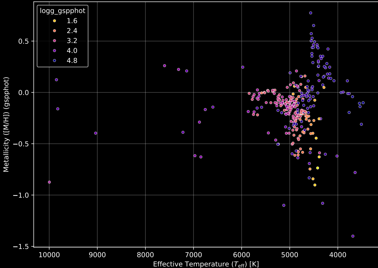
APOGEE DR17 Field: [186+31_btx] Stellar Population Parameters (n= 304)
